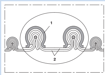
Hochtemperaturschlauch, Klemmprofilschlauch, (bis +500°C)
