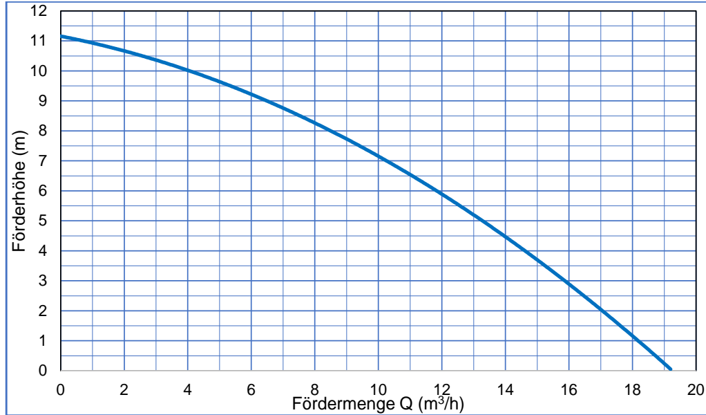
D-DWP Kennlinie
