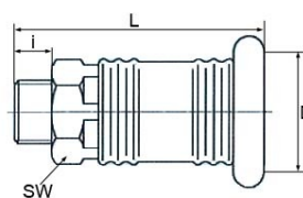
Außengewinde
