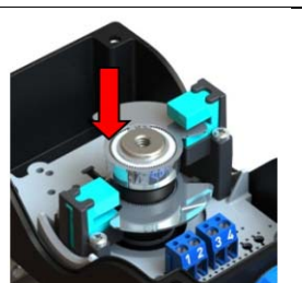
Abb. 3: Schlitz-Betätiger
